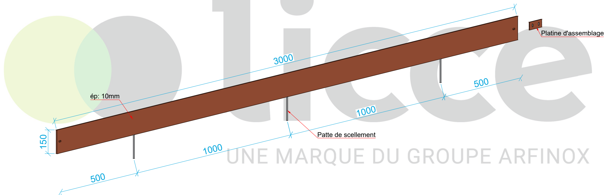
Platine d'assemblage
