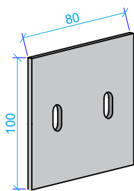
Platine d'assemblage
