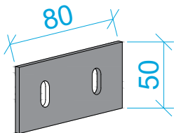
Platine d'assemblage
