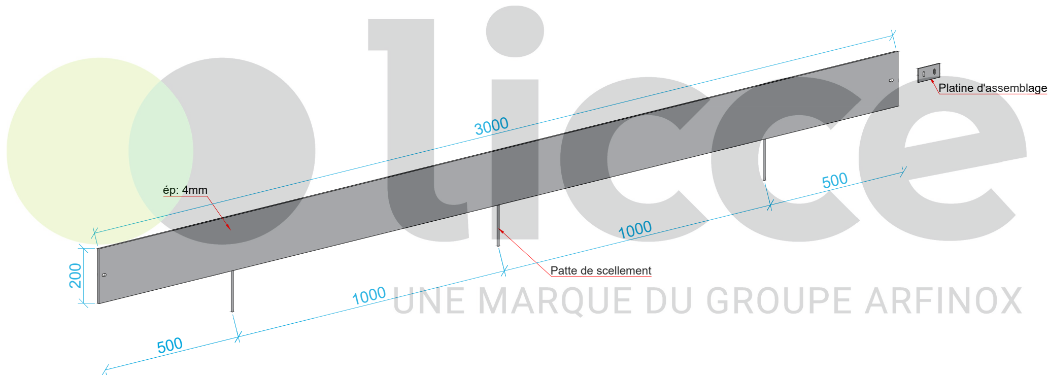
Platine d'assemblage
