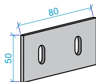
Platine d'assemblage
