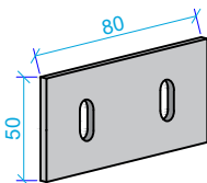
Platine d'assemblage
